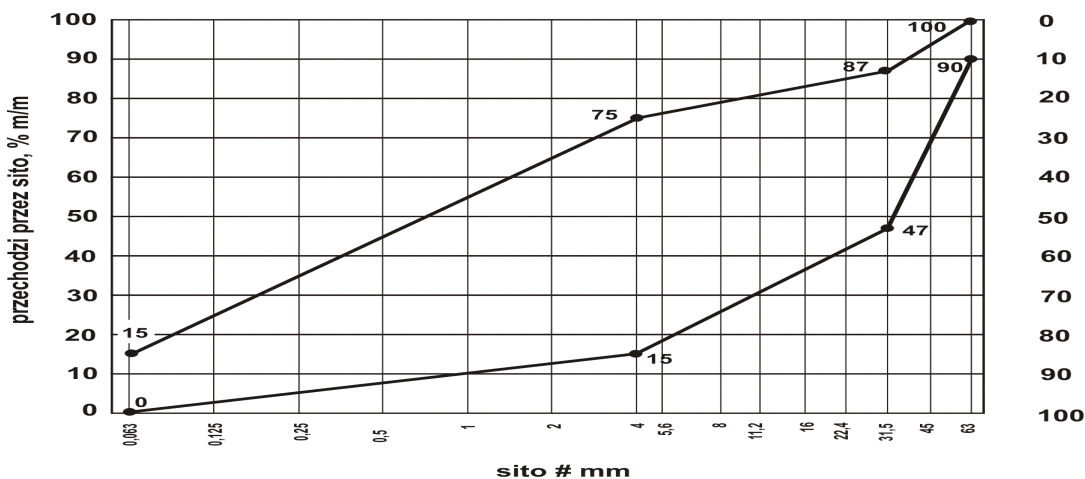
Rys. 7. Uziarnienie mieszanki niezwiązanej 0/63 dla warstwy mrozochronnej
