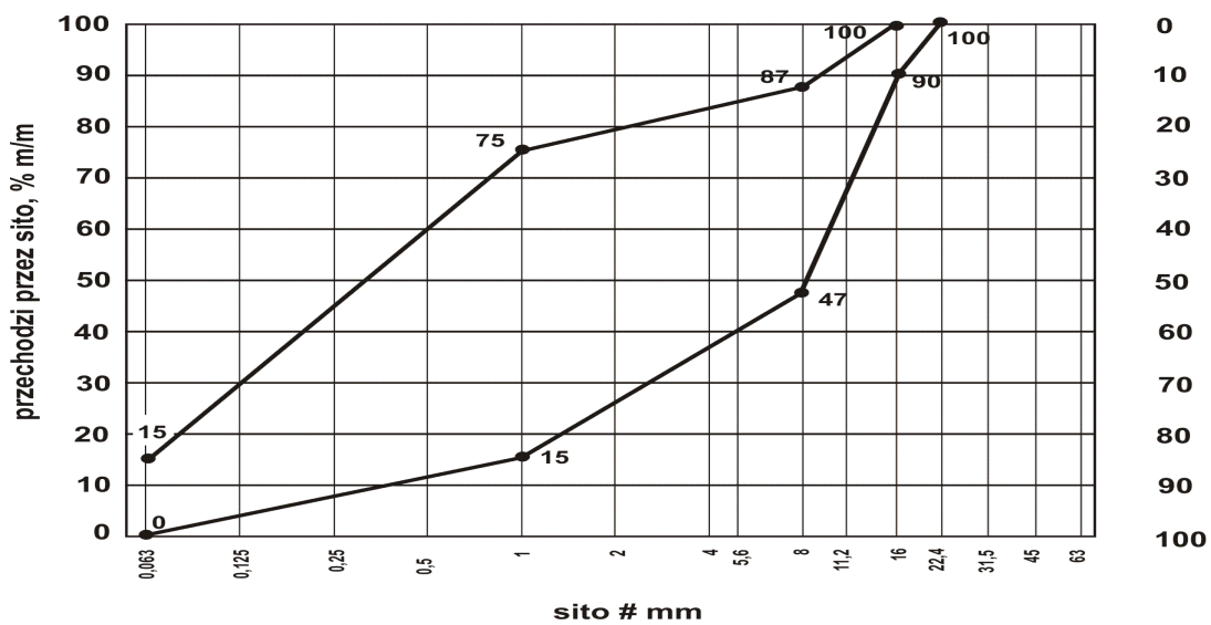
Rys. 3. Uziarnienie mieszanki niezwiązanej 0/16 dla warstwy mrozochronnej
