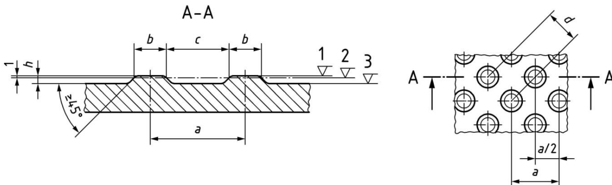
Rys. 1a. Płytki ostrzegawcze – szczegóły powierzchni
