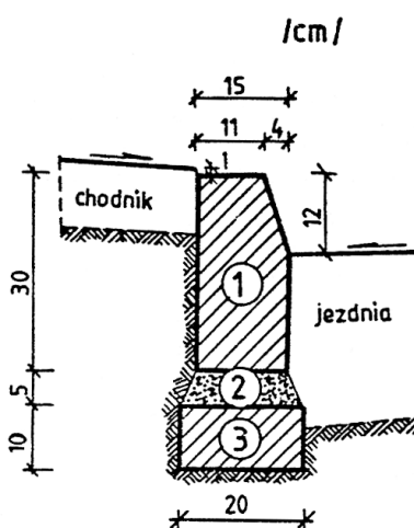
b) Krawężnik typu ulicznego 15 x 30 cm
