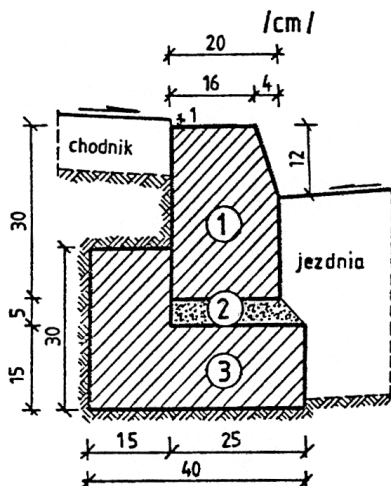
a) Krawężnik typu ulicznego 20 x 30 cm
