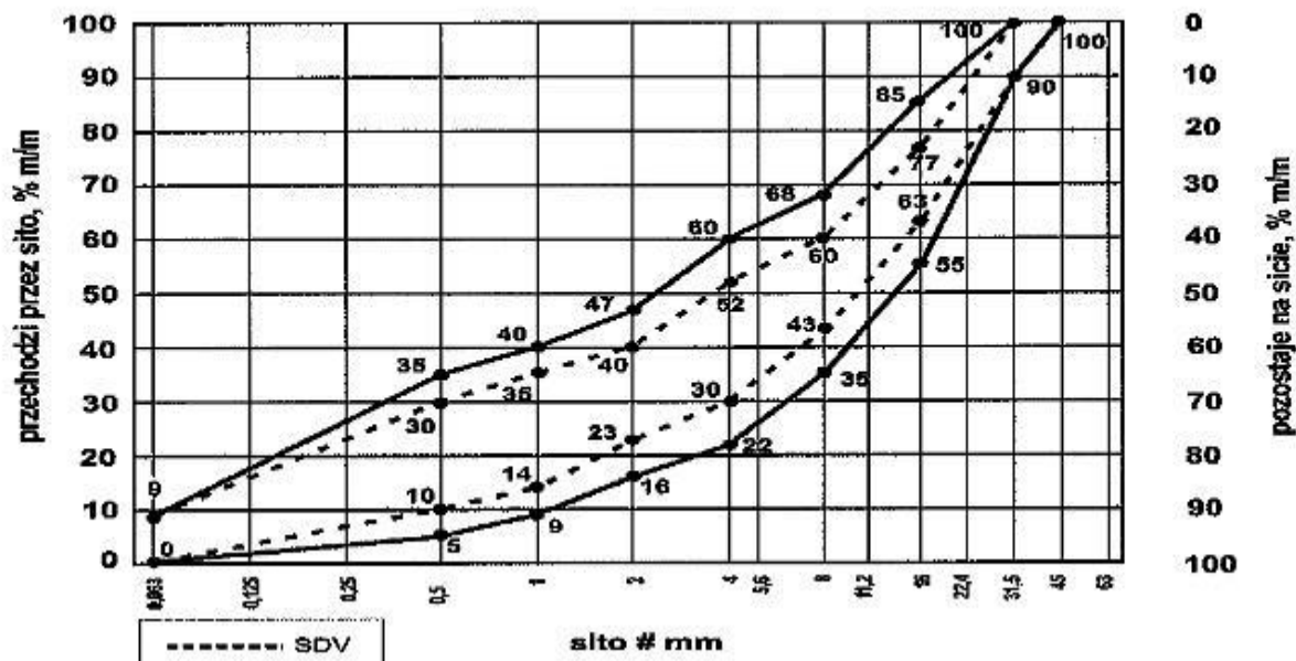
Rys. 1 Mieszanka kruszyw 0/31,5 do podbudowy zasadniczej
